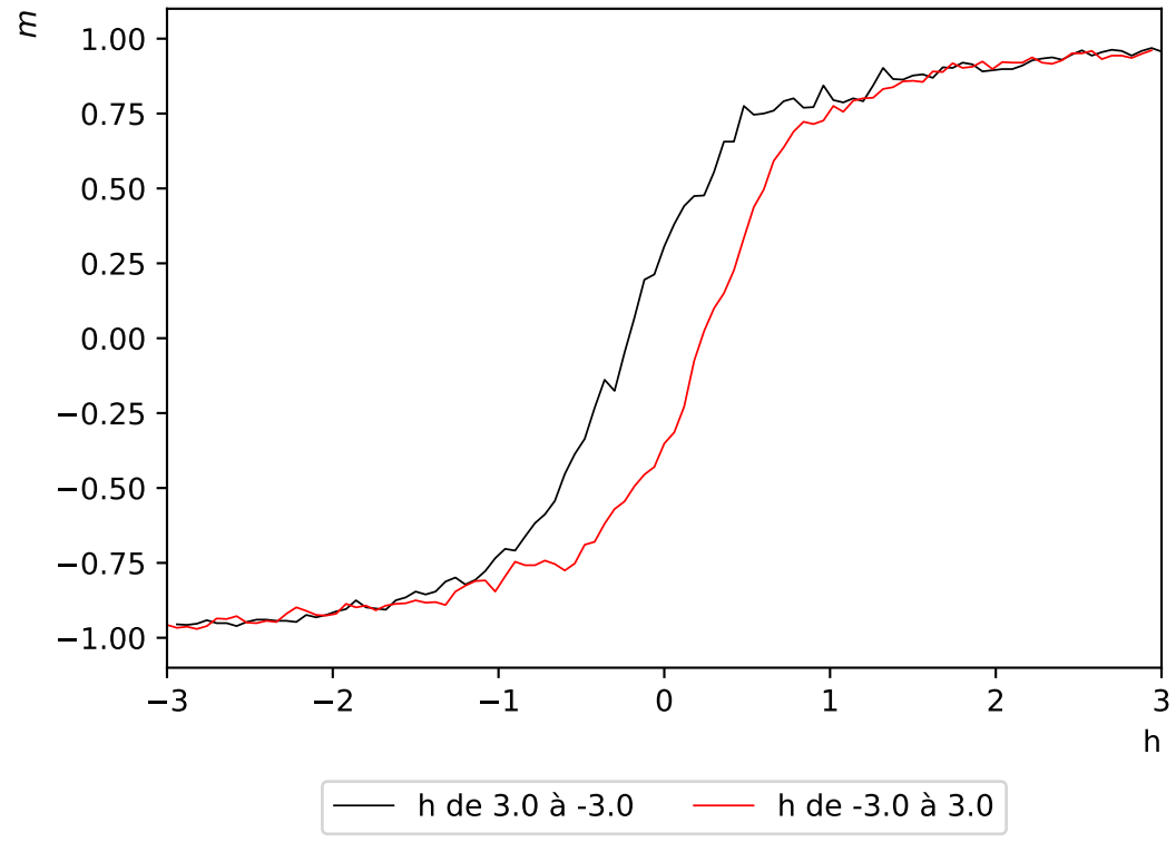
Hystérésis de l'aimantation - réseau de taille L=32 - champ magnétique d'amplitude h=3 à T=3.5
